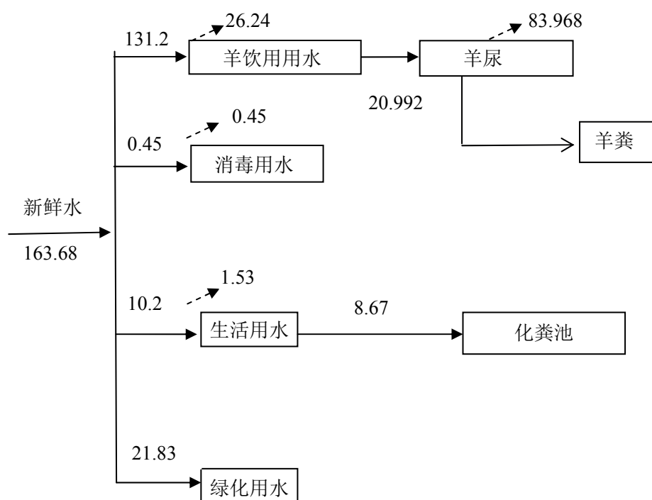
图 3.3-1 项目水平衡图 ( \text{m}^3/\text{d} )
