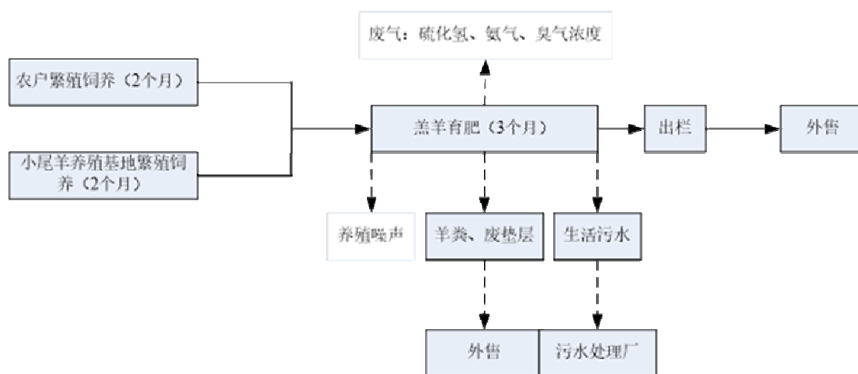
图 3.4-2 建设项目工艺流程图
