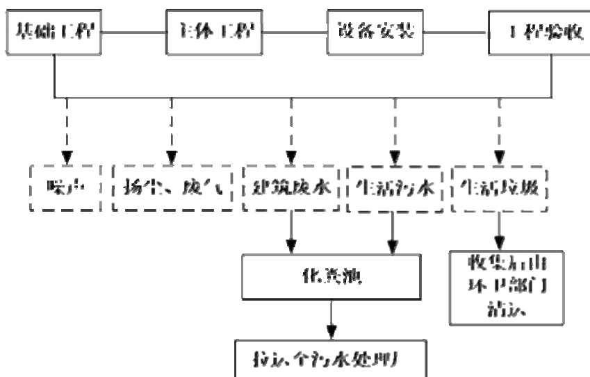
图 3.4-1 施工期工艺流程及排污节点图
