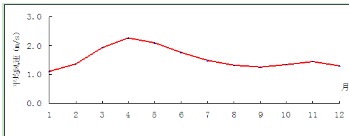
图 6.1-2 年平均风速的月变化曲线图（1988~2017 年）
