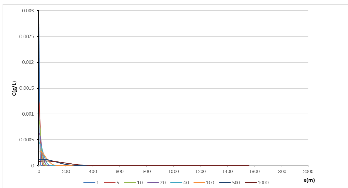
图 6.2-3 事故状况下 1000 天后氨氮浓度变化规律图
