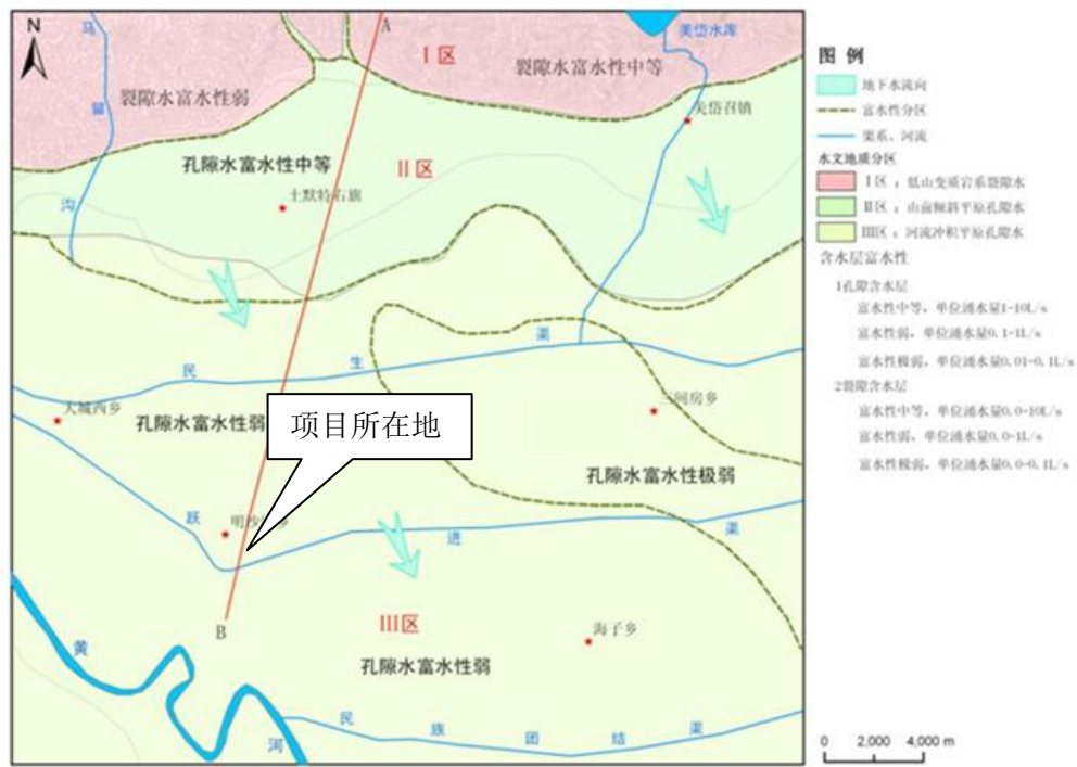
图 6.2-1 区域水文地质平面图
