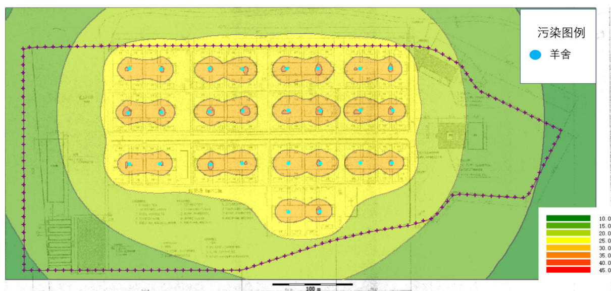
图 6.3-2 一号牧场夜间噪声预测等值线图
